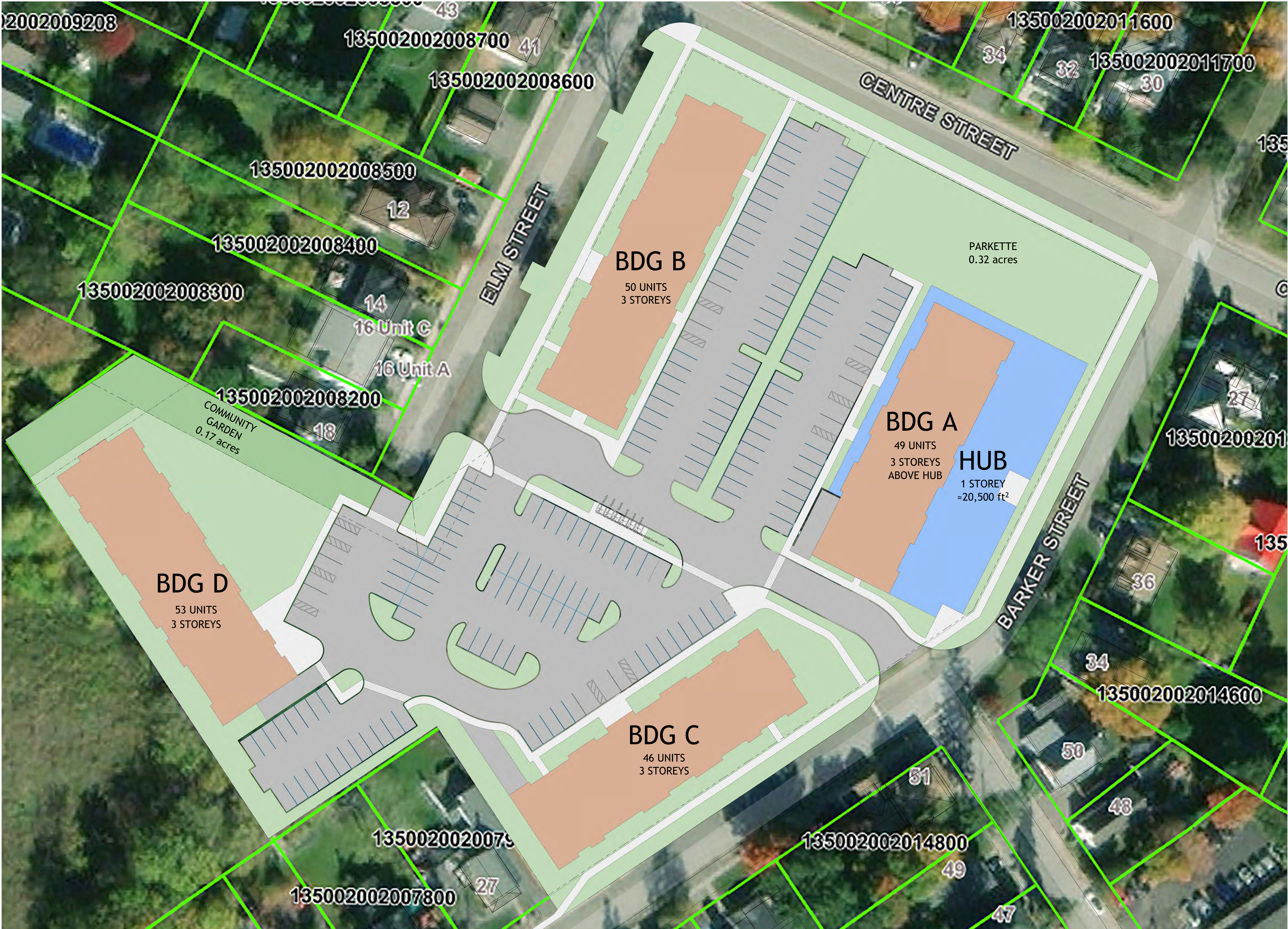
1 Site Plan 1 : 250
